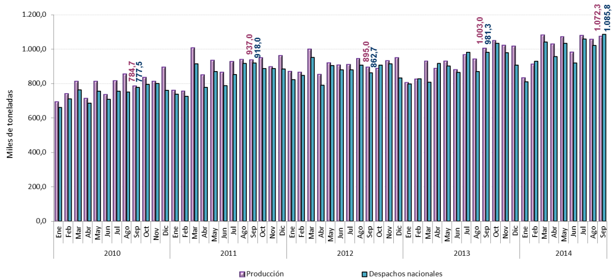
Gráfico 1 Producción y despachos mensuales de cemento gris Total nacional 2010 (enero) – 2014 (septiembre) P
