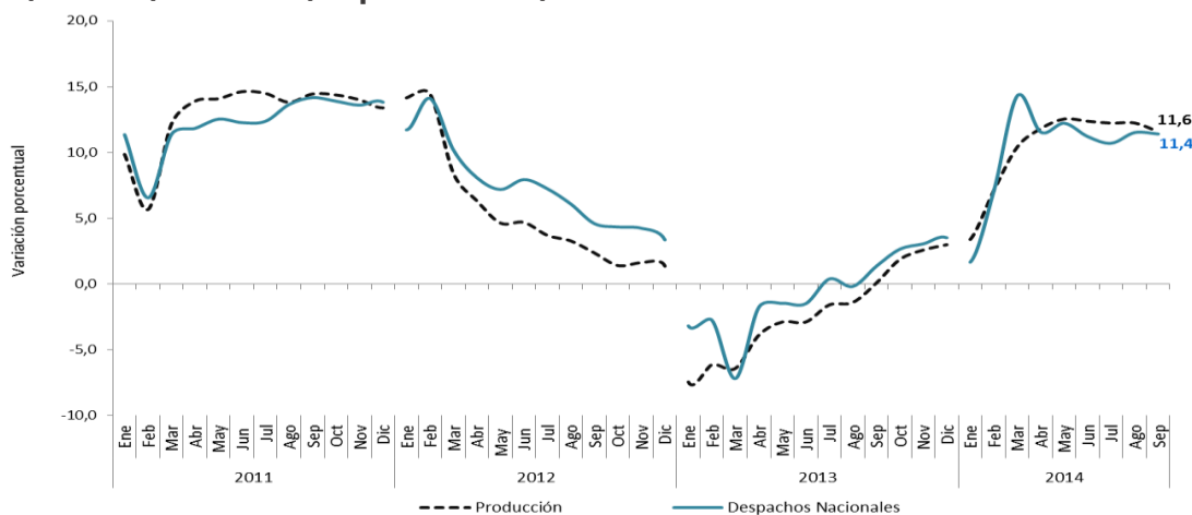
Gráfico 4 Variación año corrido de la producción y los despachos nacionales de cemento gris Total nacional 2011 (enero) - 2014 (septiembre) P
