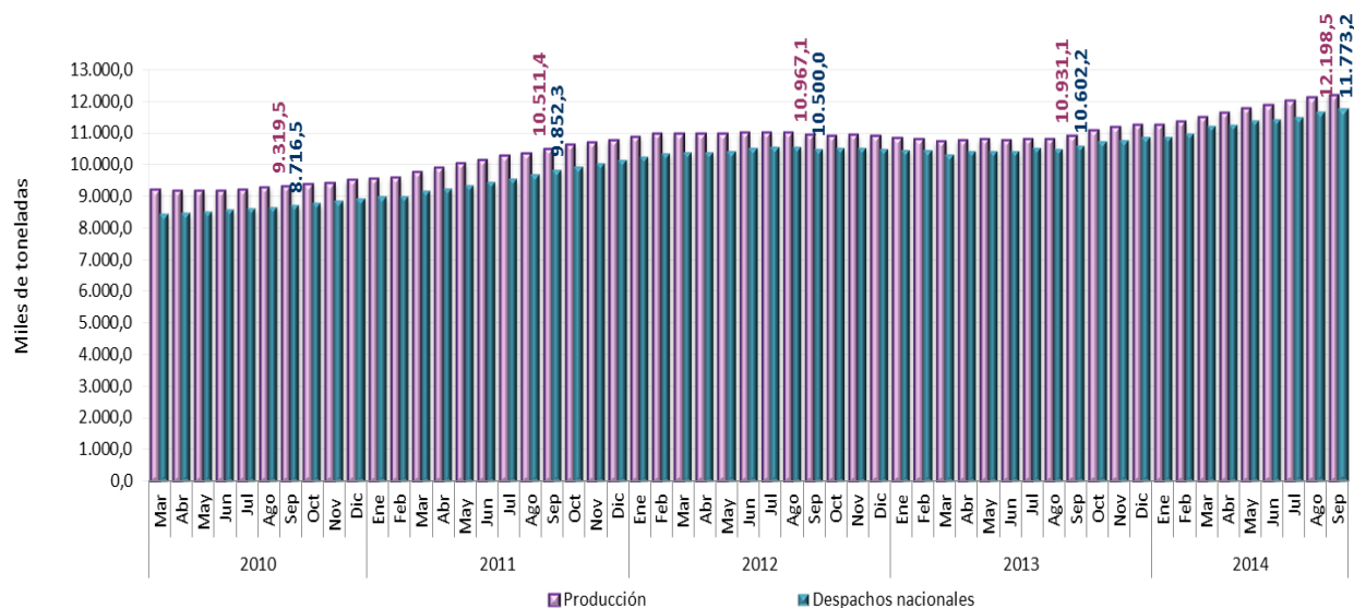
Gráfico 5 Producción y despachos nacionales de cemento gris Acumulados móviles de doce meses Total nacional 2010 (marzo) – 2014 (septiembre) P
