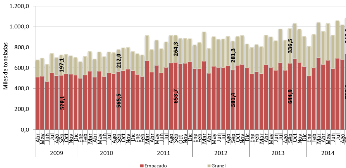
Gráfico 18 Despachos de cemento gris por tipo de empaque Total Nacional 2009 (abril) - 2014 (septiembre) P
