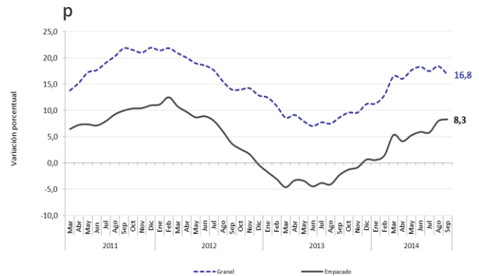
Gráfico 23 Variación acumulados móviles de doce meses de los despachos nacionales de cemento gris por tipo de empaque - Total Nacional 2011 (marzo) – 2014 (septiembre)
