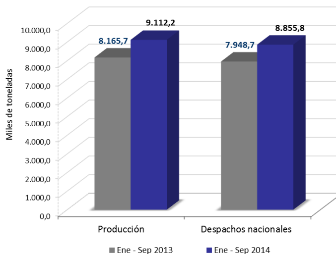
Gráfico 3 Producción y despachos nacionales de cemento gris Total nacional Enero - septiembre (2013-2014) P
