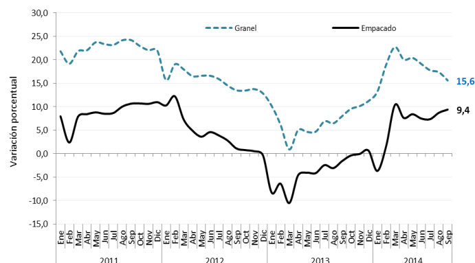
Gráfico 21 Variación año corrido de los despachos nacionales de cemento gris por tipo de empaque Total Nacional Enero – septiembre ( 2011/2014) P
