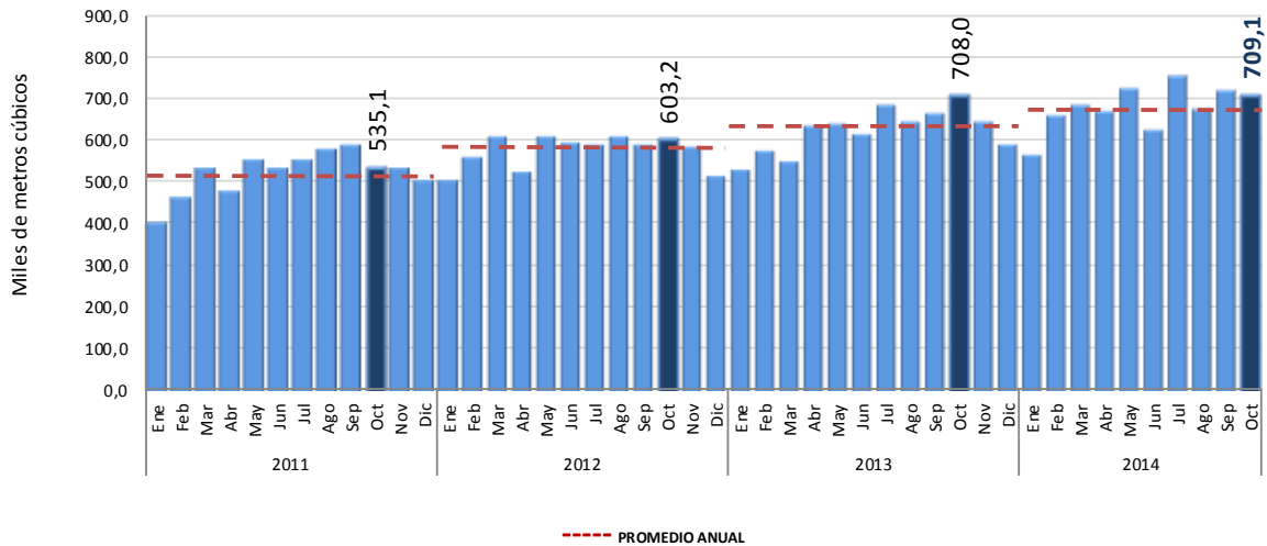
Gráfico 1 Concreto producido por la industria Total nacional 2011 – 2014 (octubre) P
