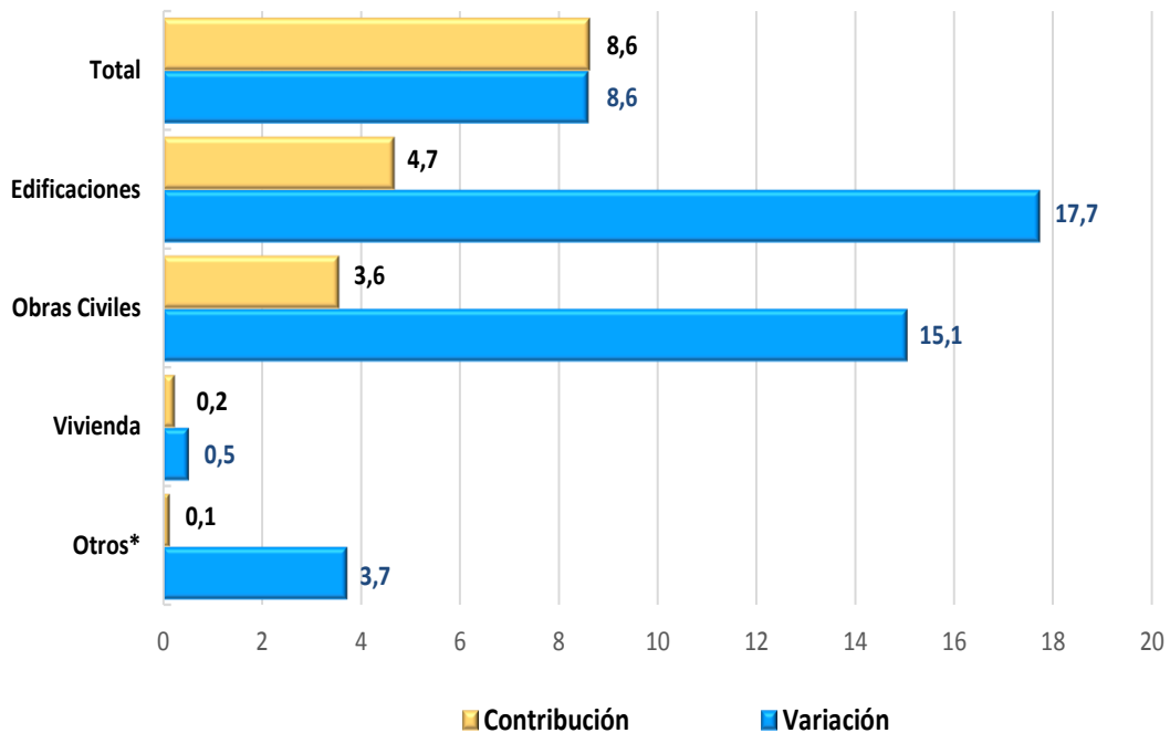
Gráfico 10 Variación año corrido del concreto producido por la industria Total nacional Enero – octubre 2014 P
