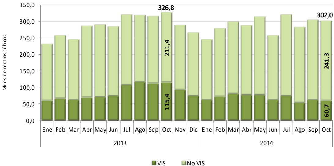
Gráfico 13 Concreto producido por la industria para vivienda (VIS y No VIS) Total nacional 2013 – 2014 (Octubre) P
