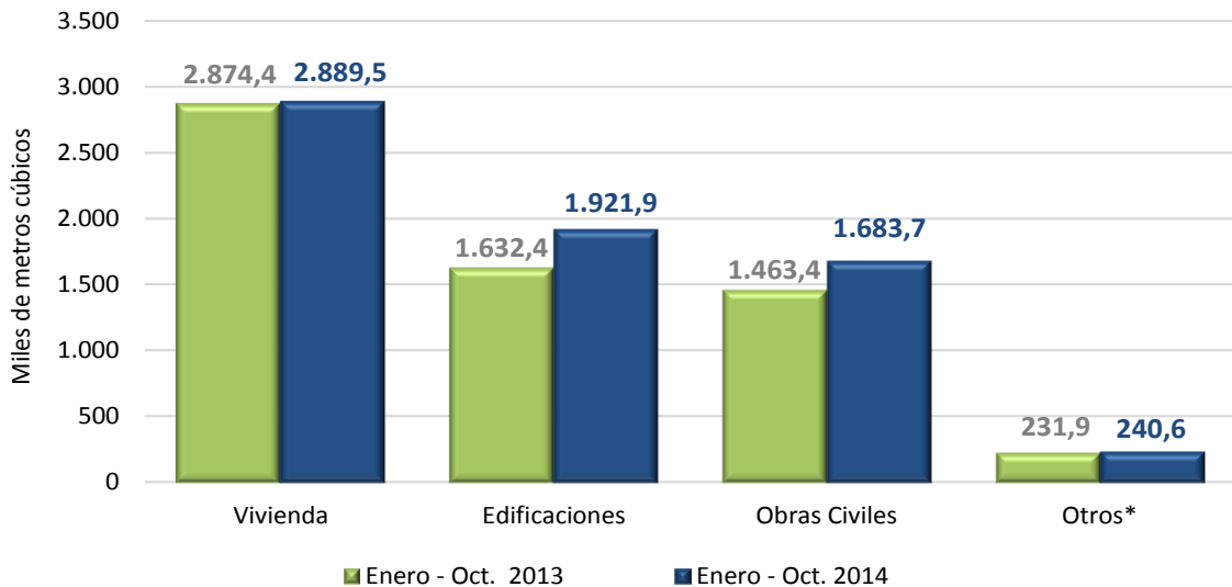
Gráfico 9 Concreto producido por la industria, según destino Total nacional Enero – octubre 2014/2013 P
