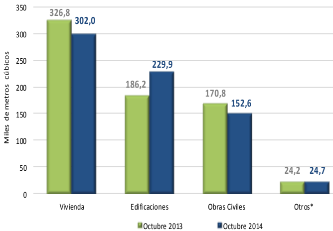
Gráfico 7 Concreto producido por la industria según destino Total nacional octubre 2014/2013 P
