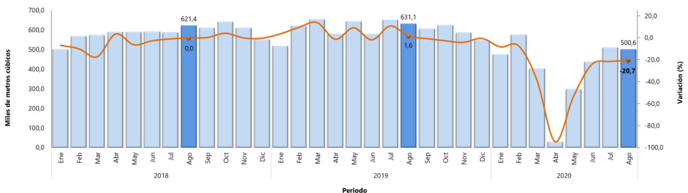
Gráfico 2. Producción de concreto premezclado (miles de metros cúbicos y variación anual) Total nacional Enero 2018 – agosto 2020 P
