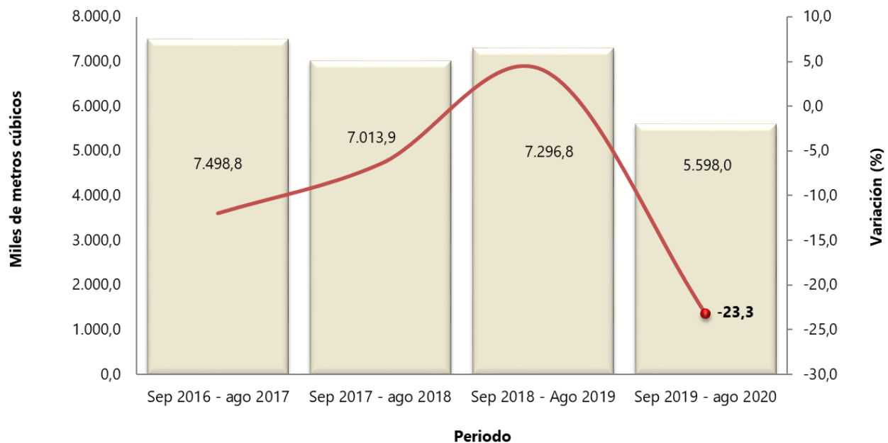
Gráfico 4. Producción de Concreto premezclado (miles de metros cúbicos y variación doce meses) Total nacional 2016 (septiembre) – 2020 P (agosto)
