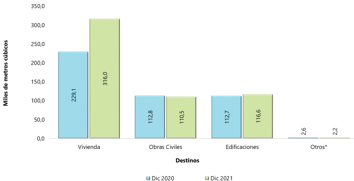
Gráfico 1. Producción de concreto premezclado según destinos (miles de metros cúbicos) Total nacional Diciembre (2020 - 2021 P )
