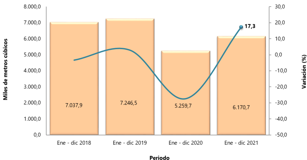
Gráfico 5. Producción de Concreto premezclado (miles de metros cúbicos y variación año corrido) Total nacional Enero - diciembre (2018 – 2021 P )
