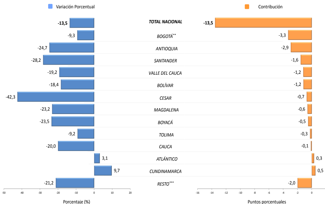
Gráfico 21. Variación doce meses del concreto premezclado, según departamentos Julio 2016 - junio 2017 P / julio 2015 - junio 2016
