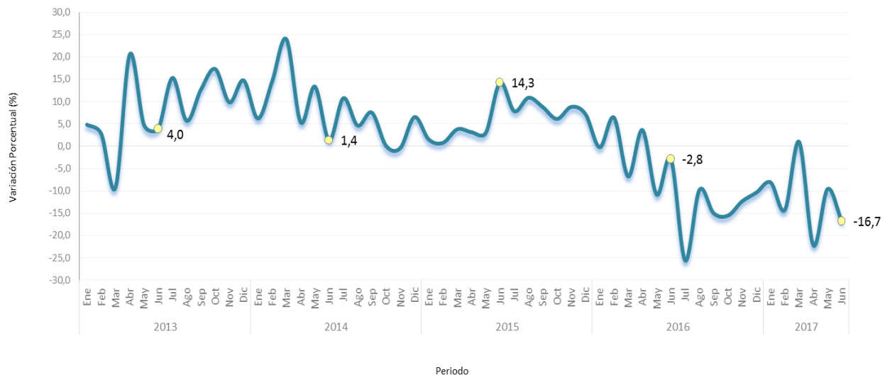
Gráfico 2. Variación anual del concreto premezclado Total nacional 2013(enero) – 2017 (junio) P
