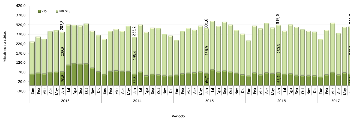
Gráfico 13. Producción concreto premezclado para vivienda (VIS y No VIS) Total nacional 2013 (enero) – 2017 (junio) P
