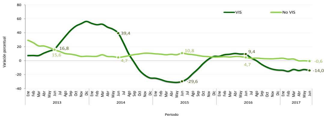
Gráfico 18. Variación doce meses del concreto premezclado para vivienda (VIS y No VIS) Julio 2016 – junio 2017 p / julio 2015 – junio 2016
