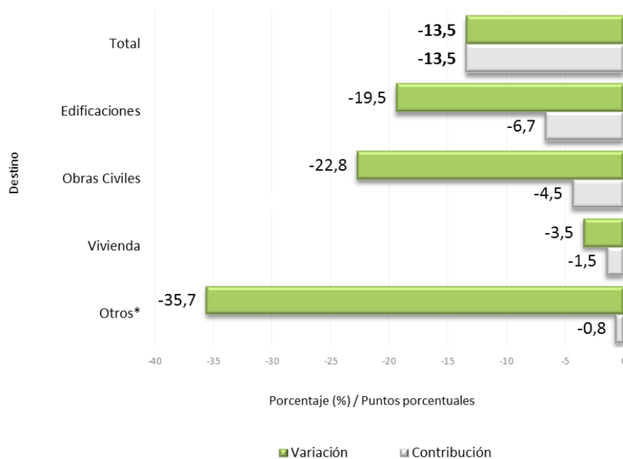
Gráfico 12. Variación y contribución doce meses del concreto premezclado, según destino Total nacional Julio 2016 – junio 2017 p / julio 2015 – junio 2016
