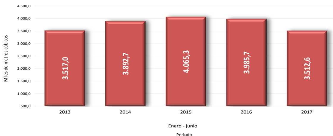
Gráfico 3. Concreto premezclado en lo corrido del año Total nacional 2013 – 2017 (enero – junio) P
