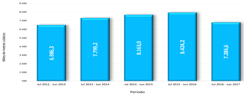
Gráfico 5. Concreto premezclado en periodos acumulados doce meses Total nacional 2012 (Julio) – 2017 (junio) P
