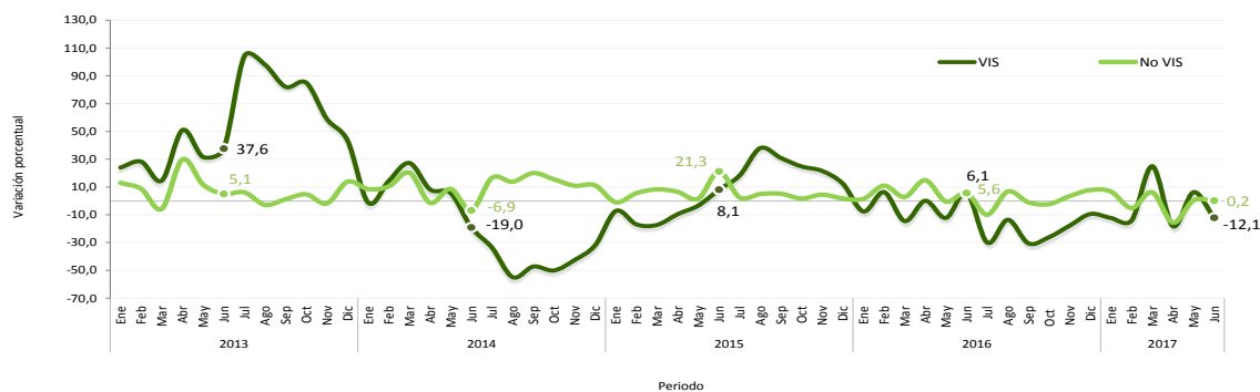
Gráfico 14. Variación anual del concreto premezclado para vivienda (VIS y No VIS) Total nacional 2013 (enero) – 2017 (junio) P
