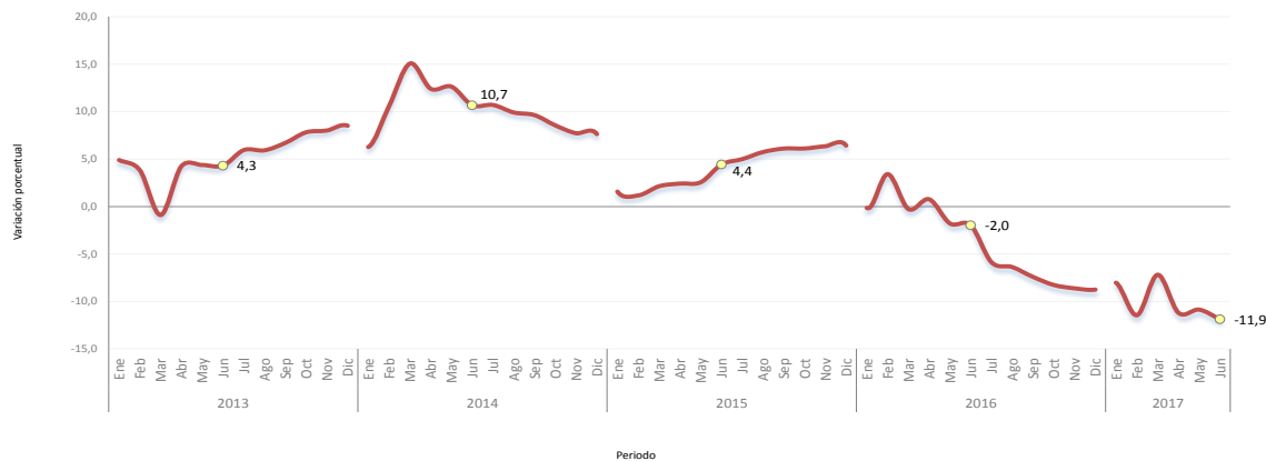
Gráfico 4. Variación año corrido del concreto premezclado Total nacional 2013 (enero) – 2017 (junio) P
