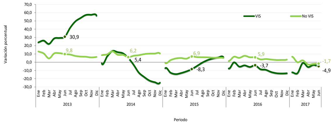
Gráfico 16. Variación año corrido del concreto premezclado para vivienda (VIS y No VIS) 2013 (enero) - 2017 p (junio)
