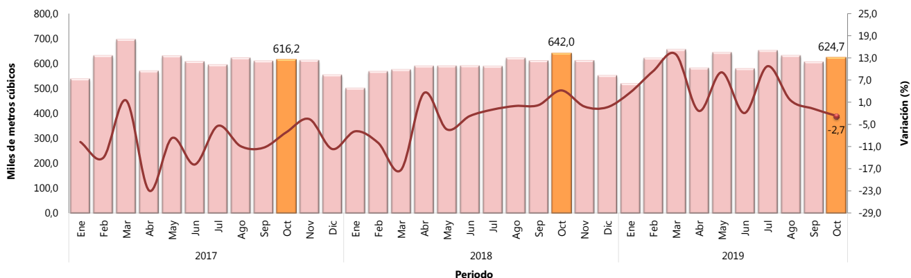
Gráfico 2. Producción de concreto premezclado (miles de metros cúbicos / variación anual) Total nacional 2017 (enero) – 2019 P (octubre)
