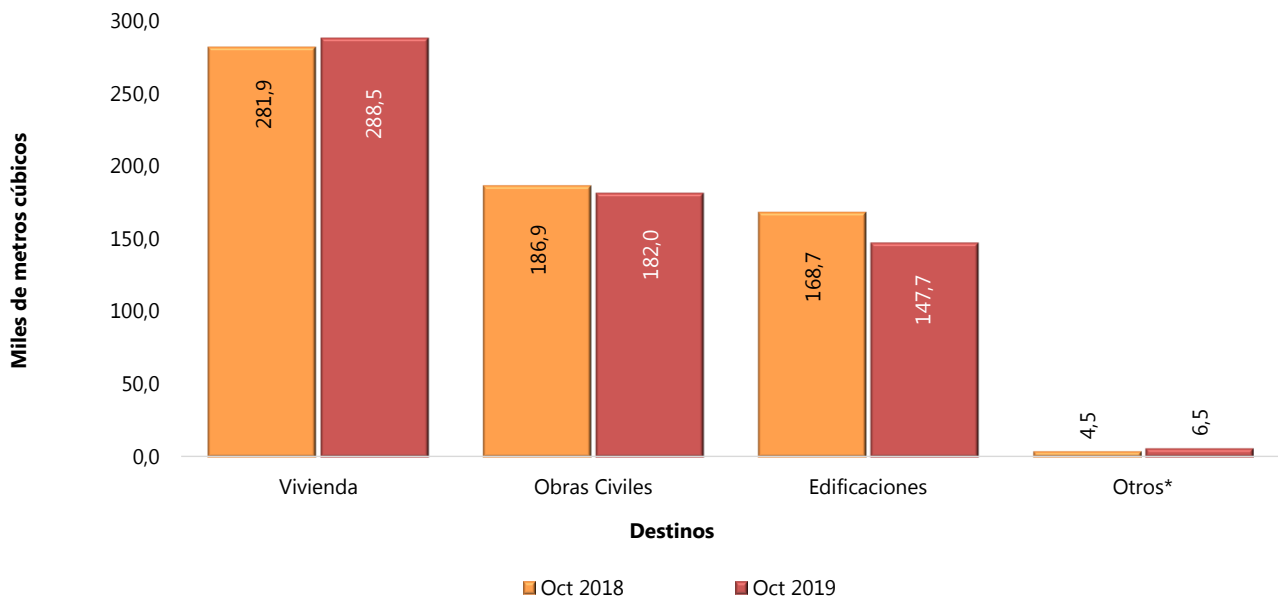
Gráfico 1. Producción de concreto premezclado según destinos (miles de metros cúbicos) Total nacional Octubre (2018 - 2019 P )
