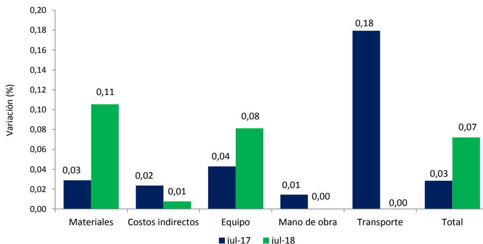
Variación mensual del Índice de costos de la construcción pesada (ICCP), por grupos de costo 2017-2018 (julio)
