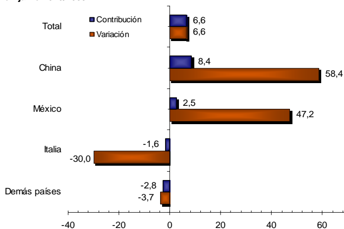
Gráfico 20 Comportamiento del valor CIF de las importaciones de calderas, máquinas y partes Total nacional Enero - junio 2010/2009
