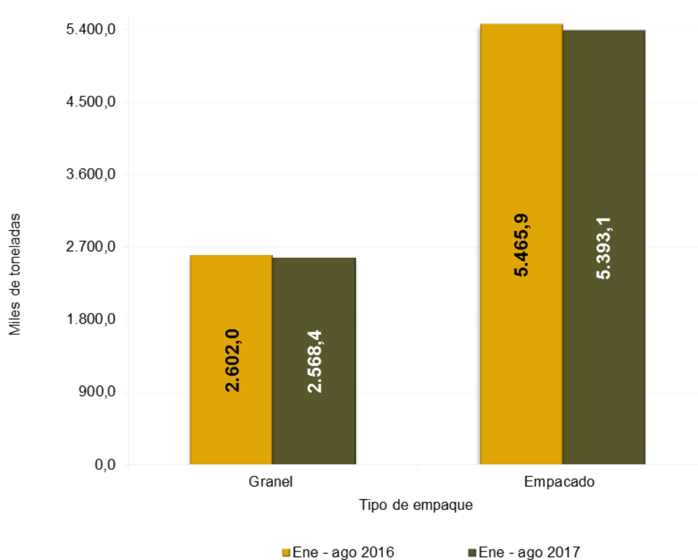
Gráfico 20. Despachos nacionales de cemento gris, según tipo de empaque Total Nacional Enero – agosto 2017 p / 2016
