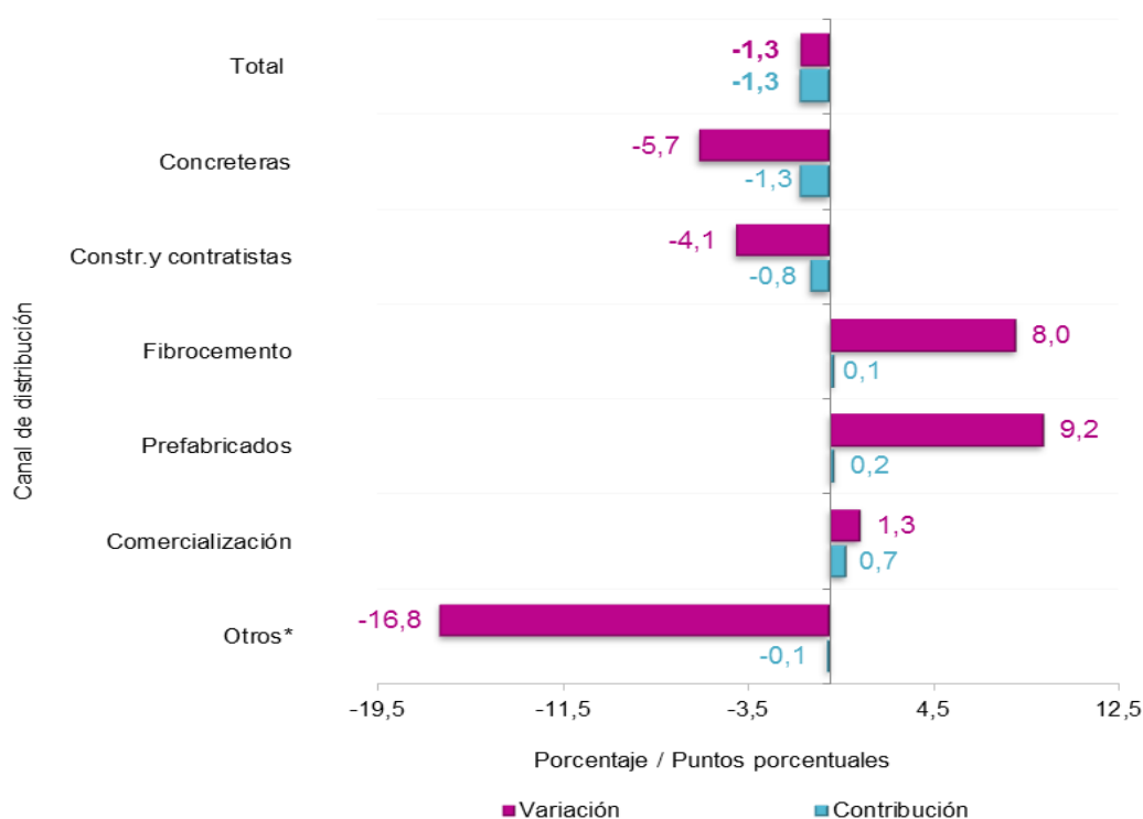
Gráfico 10. Variación y contribución año corrido de los despachos de cemento gris, según canal de distribución Total Nacional Enero – agosto 2017 P / 2016
