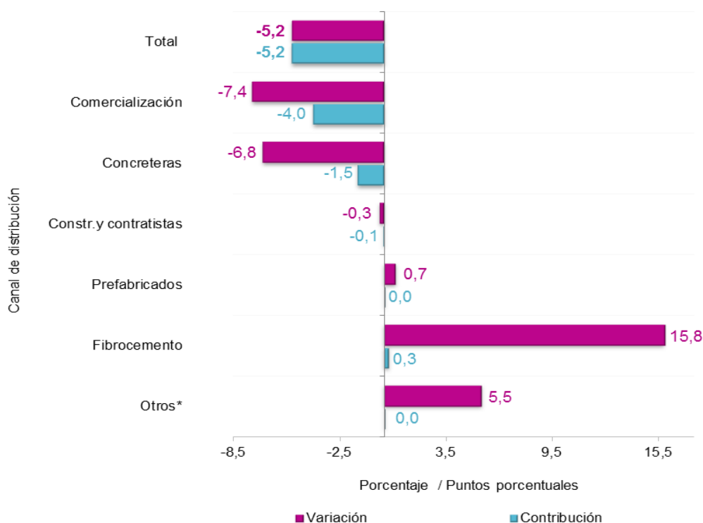
Gráfico 9. Variación y contribución anual de los despachos de cemento gris, según canal de distribución Total Nacional Agosto 2017 p / 2016
