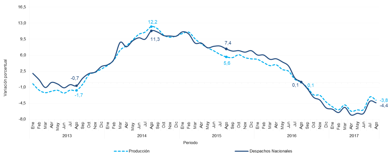
Gráfico 6. Variación acumulada doce meses de la producción y los despachos nacionales de cemento gris Total nacional 2013 (enero) – 2017 (agosto) P
