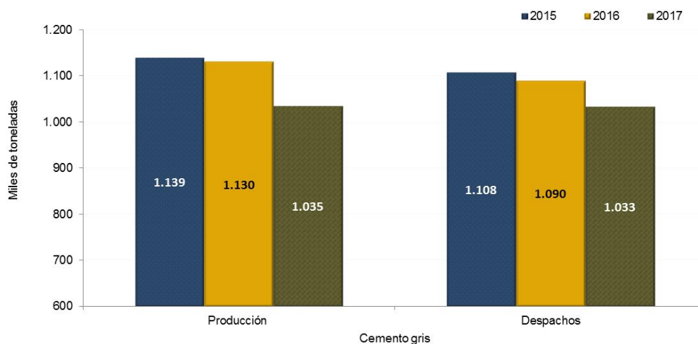
Producción y despachos de cemento gris Agosto (2015-2017 P )
