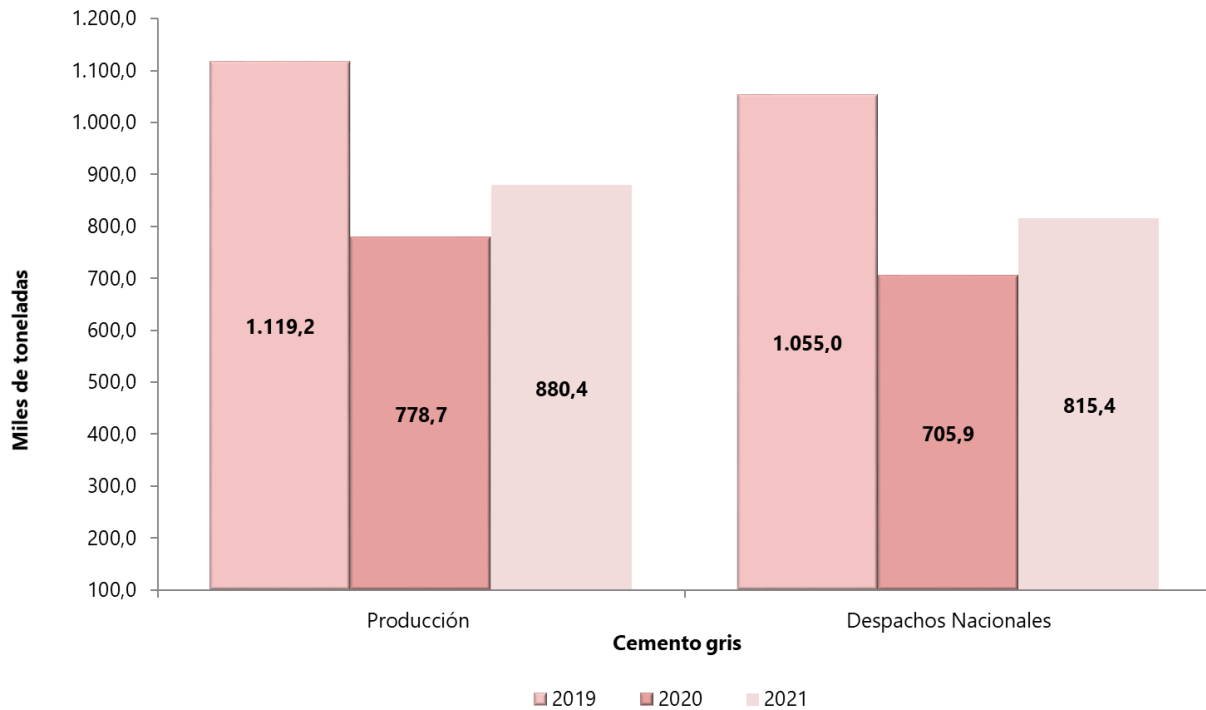
Gráfico 1. Producción y despachos de cemento gris (miles de toneladas) Total nacional Mayo (2019 – 2021 P )
