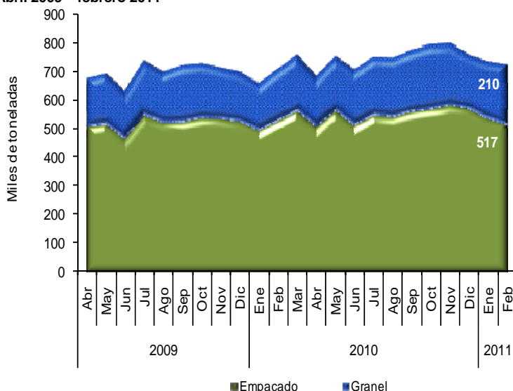
Gráfico 16 Despachos de cemento gris por tipo de empaque Total Nacional Abril 2009 – febrero 2011 P
