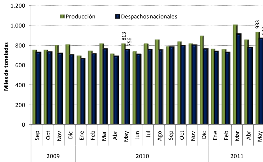
Gráfico 1 Producción y despachos mensuales de cemento gris Total Nacional Septiembre 2009 – mayo 2011 P
