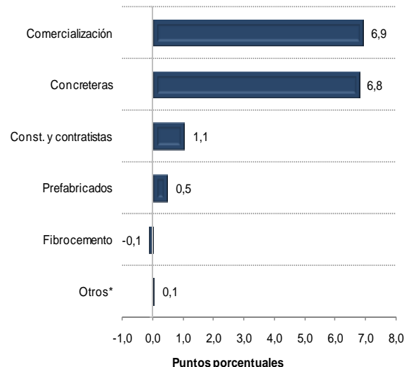
Gráfico 10 Contribución a la variación anual de despachos de cemento gris según canal de distribución Total Nacional Mayo 2011 P
