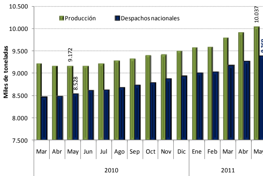
Gráfico 5 Producción y despachos nacionales de cemento gris Acumulados móviles de doce meses Total Nacional Marzo 2010 - mayo 2011 P
