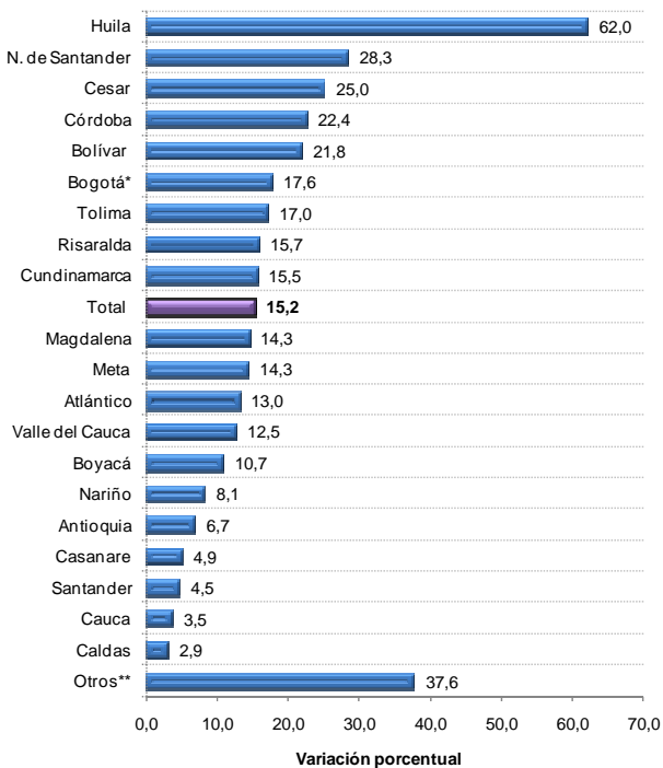
Gráfico 17 Variación anual de los despachos de cemento gris según departamento de destino Total Nacional Mayo 2011 P
