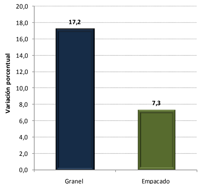
Gráfico 29 Variación acumulada doce meses de la producción y los despachos nacionales por tipo de empaque Total Nacional Junio 2010 - mayo 2011 / junio 2009 - mayo 2010
