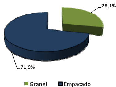
Gráfico 23 Distribución de los despachos de cemento gris por tipo de empaque Total Nacional Mayo 2011 P
