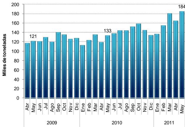
Gráfico 11 Evolución de los despachos de cemento gris por principales canales de distribución Total Nacional Abril 2009 – mayo 2011 P
