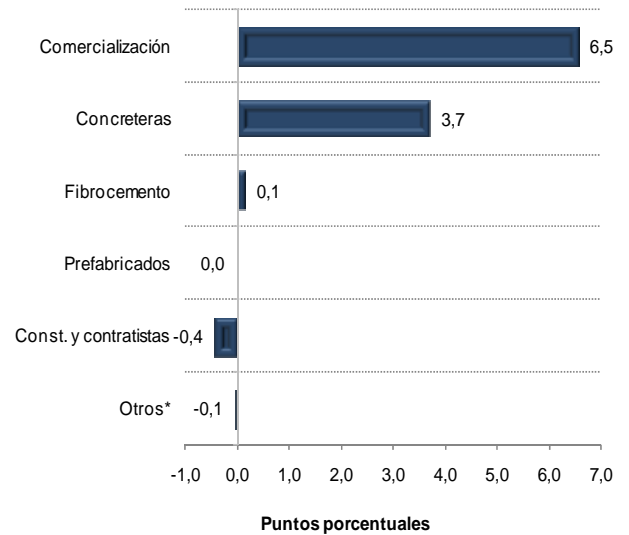
Gráfico 15 Contribución a la variación acumulada doce meses de los despachos de cemento gris según canal de distribución Total Nacional Junio 2010 – mayo 2011 P
