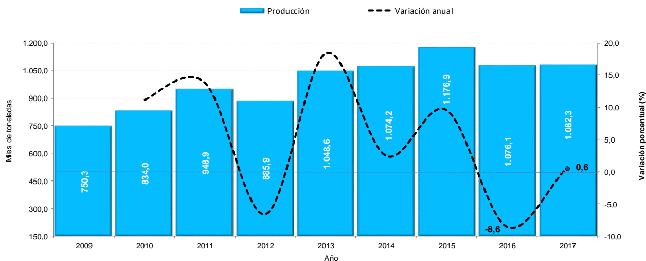
Producción de cemento gris y variación anual Total nacional Octubre (2009 – 2017)
