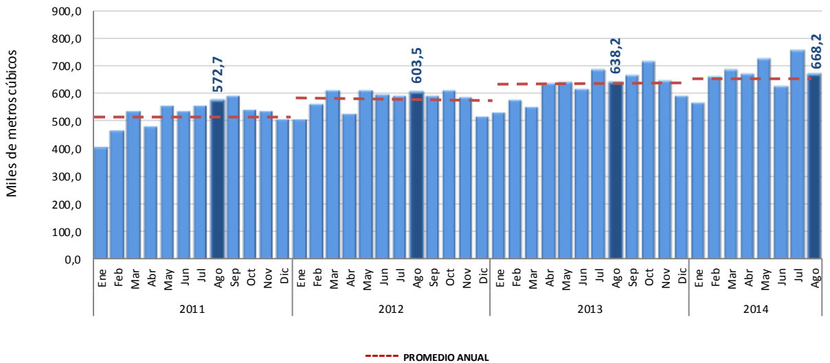
Gráfico 1 Concreto producido por la industria Total nacional 2011 – 2014 (agosto) P
