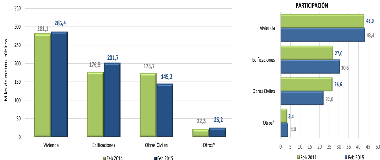
Gráfico 7 Producción concreto premezclado Total nacional Febrero 2015/2014 p
