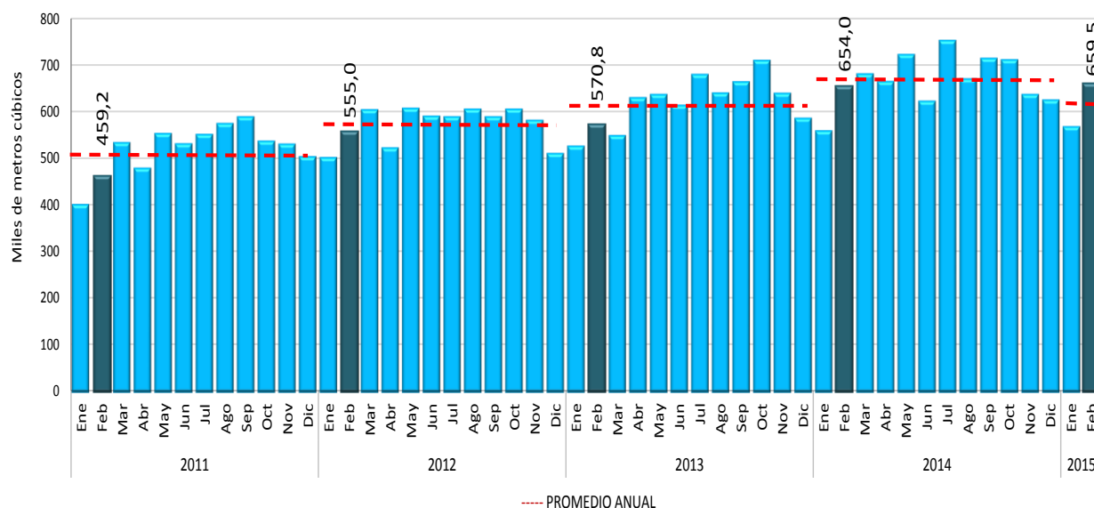
Gráfico 1 Producción concreto premezclado Total nacional 2011 – 2015 (febrero) p
