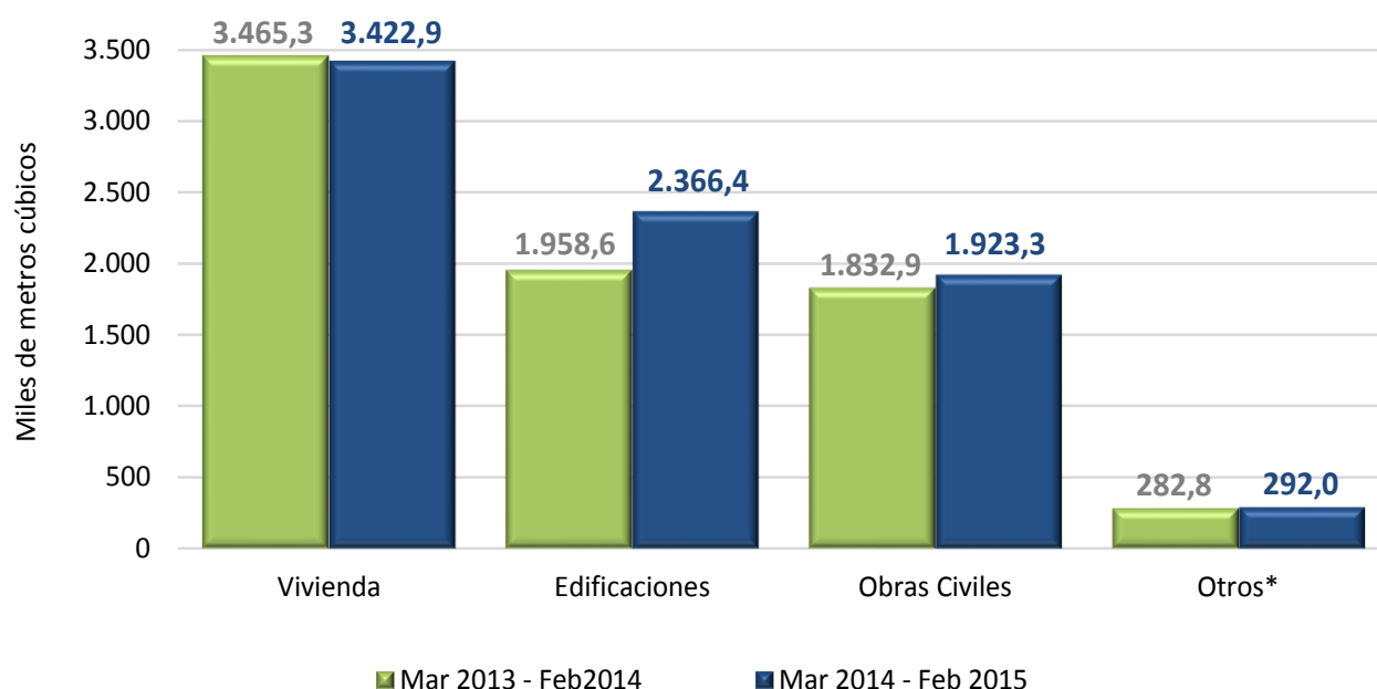
Gráfico 11 Producción concreto premezclado, según destino Total nacional Marzo 2014 - febrero 2015 / marzo 2013 - febrero 2014 p
