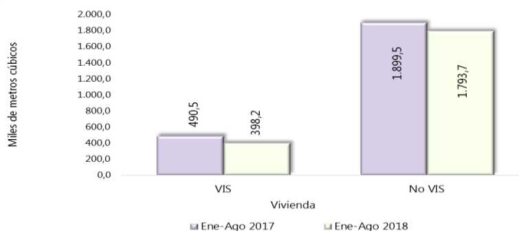
Gráfico 7. Producción año corrido de Concreto premezclado destinado a vivienda, VIS y No VIS (miles de metros cúbicos) Total nacional Enero-agosto 2018 p / enero-agosto 2017
