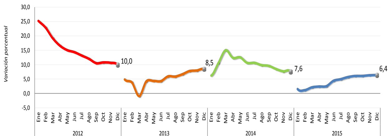
Gráfico 4 Variación acumulada doce meses del concreto premezclado Total nacional 2012 – 2015 (enero - diciembre) P
