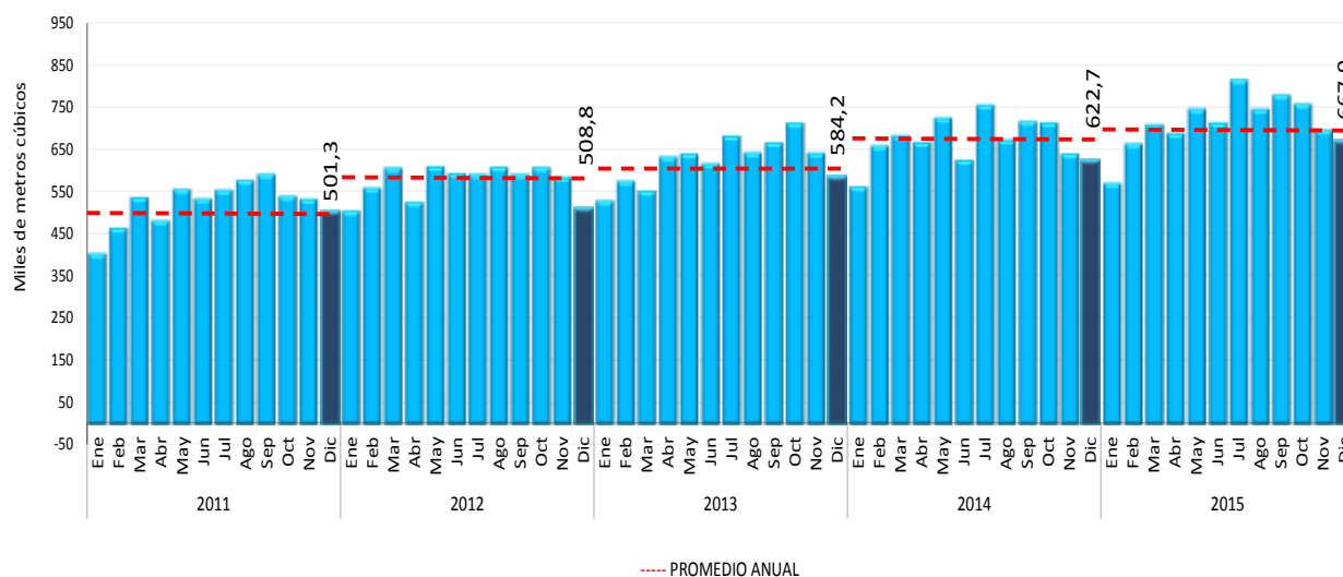
Gráfico 1 Producción concreto premezclado Total nacional 2011(enero) – 2015 (diciembre) P
