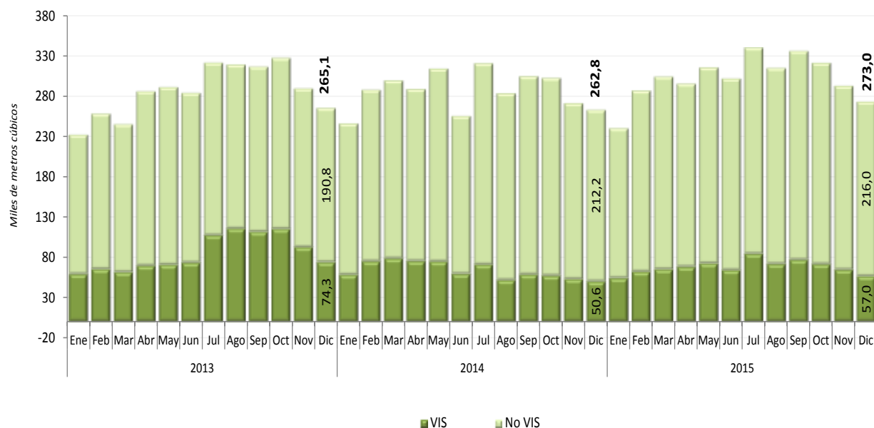
Gráfico 9 Producción concreto premezclado para vivienda (VIS y No VIS) Total nacional 2013 (enero) – 2015 (diciembre) p
