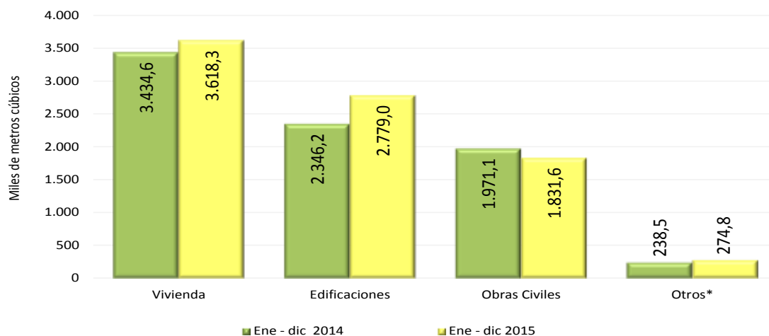
Gráfico 7 Concreto premezclado, según destino Total nacional Enero – diciembre 2015 / 2014 p
