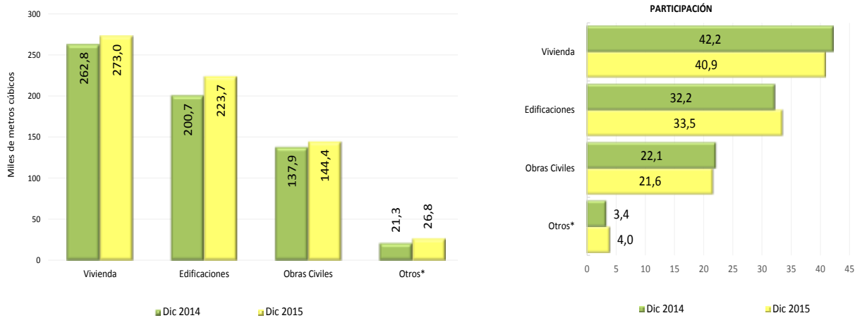
Gráfico 5 Producción concreto premezclado Total nacional Diciembre 2015/2014 p
