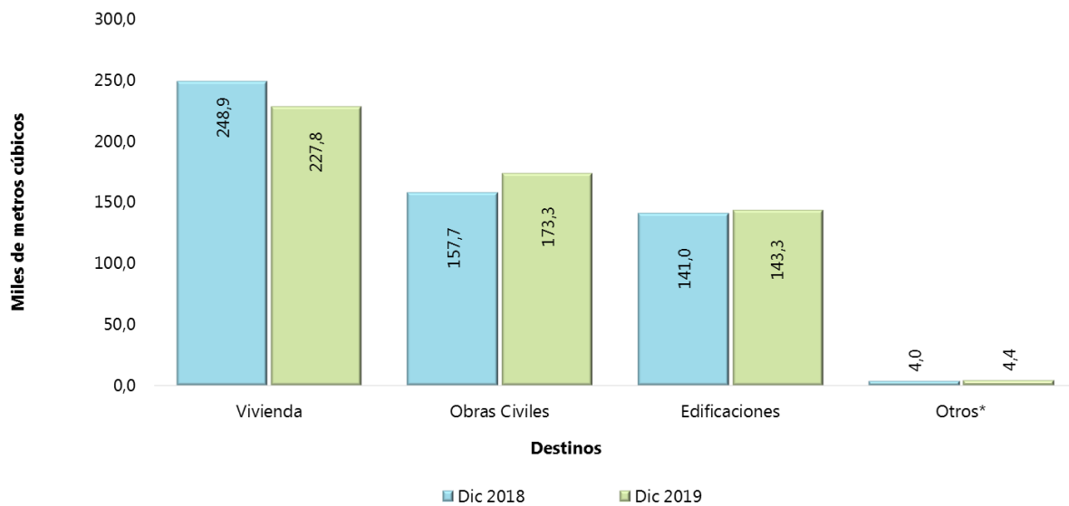
Gráfico 1. Producción de concreto premezclado según destinos (miles de metros cúbicos) Total nacional Diciembre (2018 - 2019 p )
