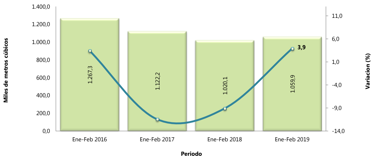
Gráfico 3. Producción de Concreto premezclado (miles de metros cúbicos / variación año corrido) Total nacional Enero - febrero (2016 –2019 P )
