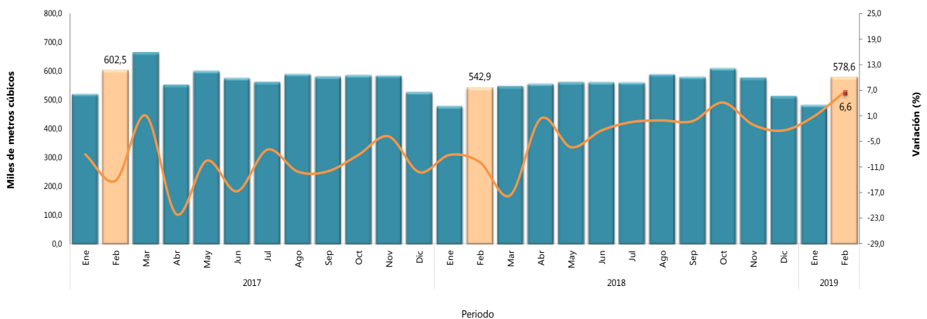
Gráfico 2. Producción de concreto premezclado (miles de metros cúbicos / variación anual) Total nacional 2017 (enero) – 2019 P (febrero)
