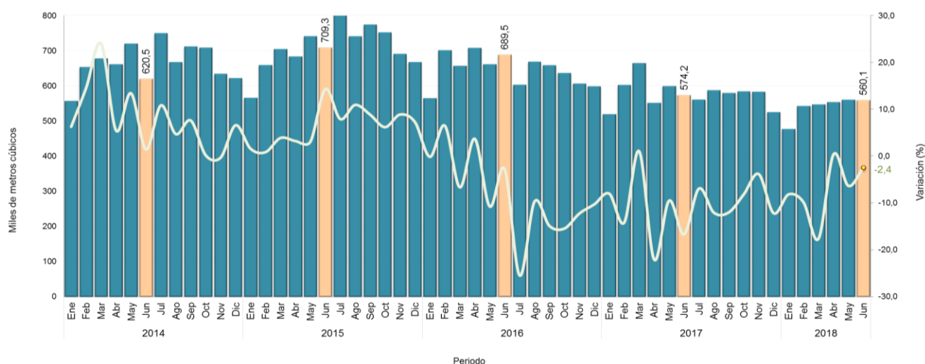
Gráfico 2. Producción anual de concreto premezclado ( miles de metros cúbicos y variación porcentual) Total nacional 2014 (enero) – 2018 (junio) p
