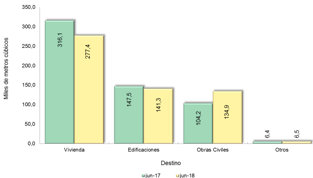
Gráfico 1. Producción de concreto premezclado según destinos (Miles de metros cúbicos) Total nacional Junio (2017 – 2018) p
