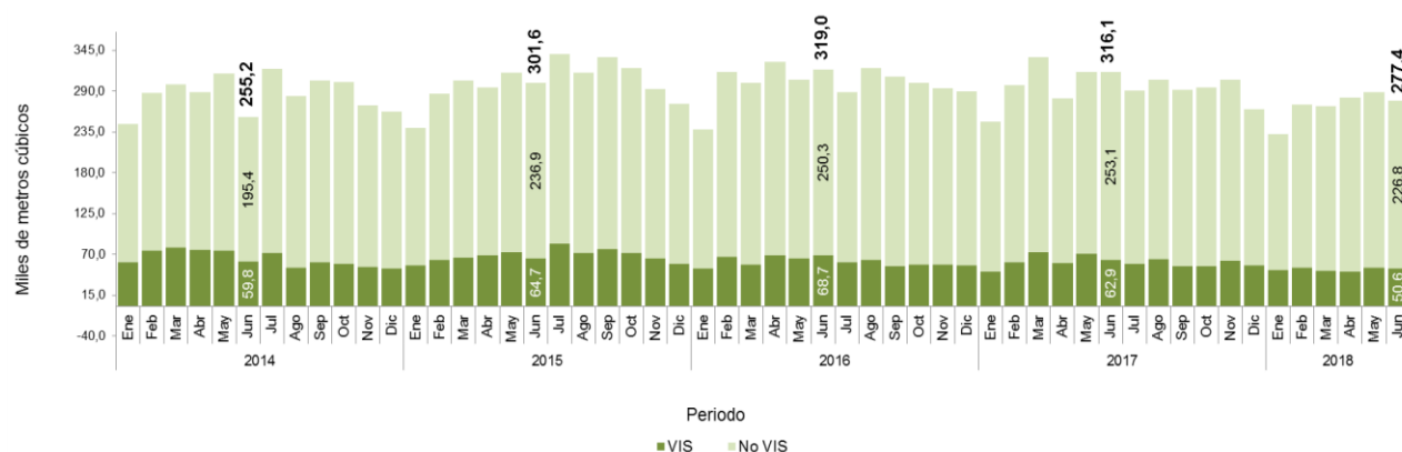
Gráfico 5. Producción concreto premezclado para vivienda, VIS y No VIS (miles de metros cúbicos) Total nacional 2014 (Enero) – 2018 (junio) p
