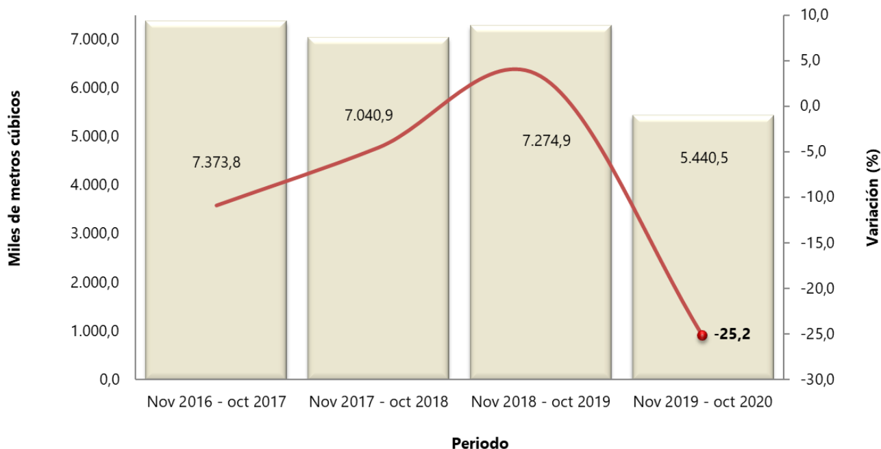
Gráfico 4. Producción de Concreto premezclado (miles de metros cúbicos y variación doce meses) Total nacional 2016 (noviembre) – 2020 P (octubre)
