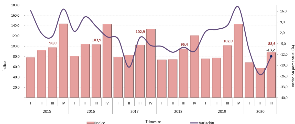
Gráfico 7. Índice y variación anual de los pagos de vías de agua, puertos, represas, acueductos, alcantarillado y otras obras portuarias Total nacional – serie empalmada 2015 – 2020 Pr (III trimestre)
