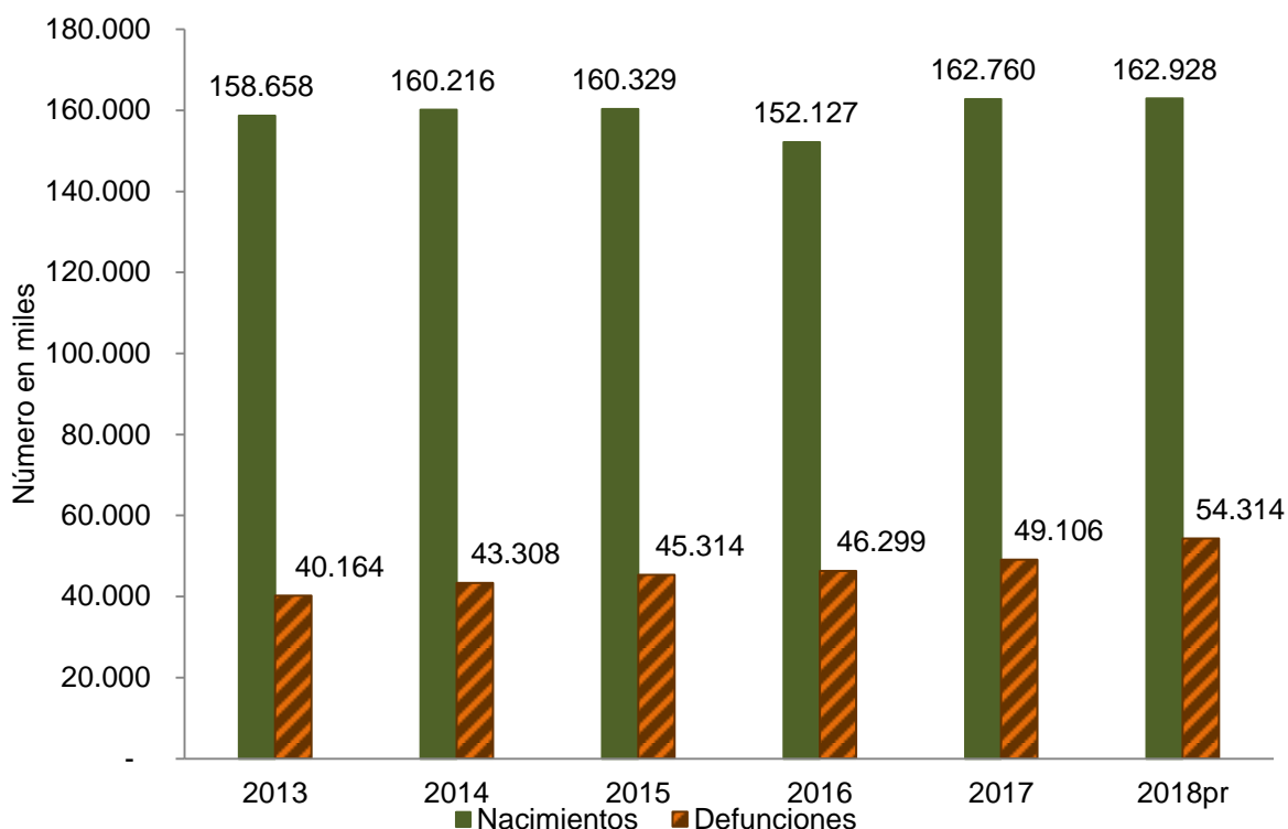
Gráfico 1. Número de nacimientos y defunciones en Colombia. Total nacional IV trimestre (2013-2018pr)
