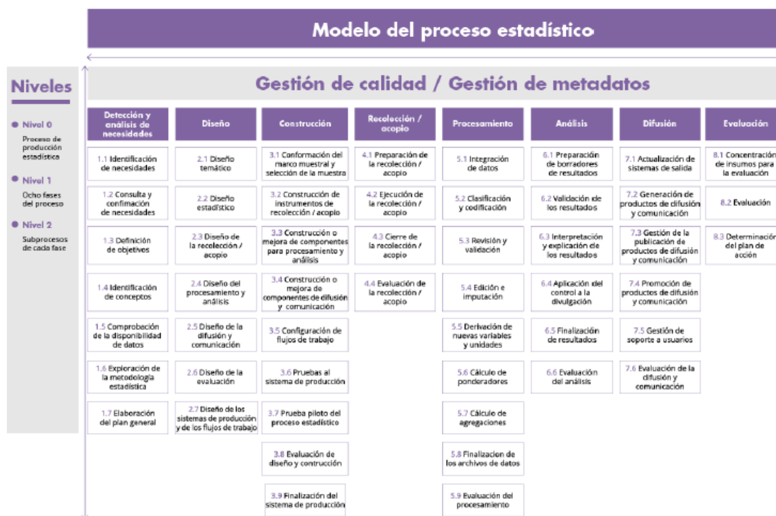
Figura 9. Modelo del proceso estadístico.
