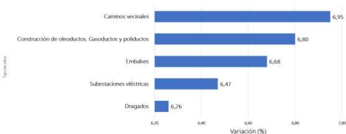
Gráfica 7. ICOCIV. Menores variaciones anuales, según tipología de obra
