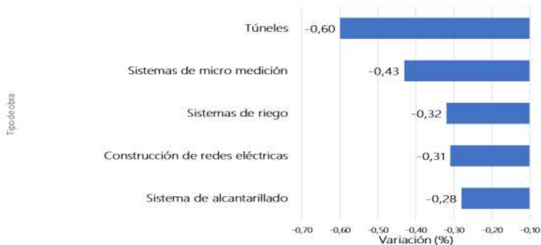
Gráfica 3. ICOCIV. Mayores variaciones mensuales negativas, según tipología de obra Total nacional Abril 2024
