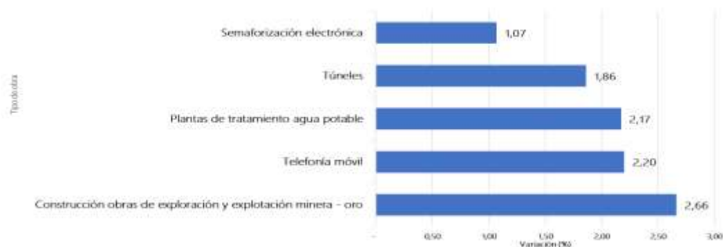
Gráfica 5. ICOCIV. Menores variaciones del año corrido, según tipología de obra Total nacional Abril 2024
