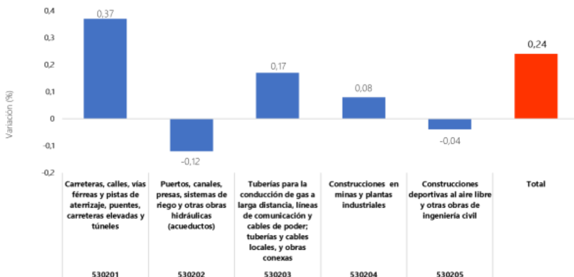
Gráfico 1. Variación mensual del ICOCIV según agrupaciones CPC v2 A.C. (%) Total, nacional Abril 2024
