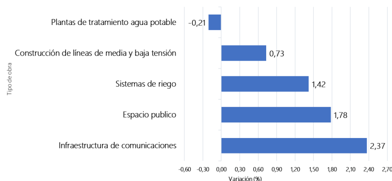
Gráfico 7. ICOCIV. Menores variaciones anuales, según tipología de obra Total nacional Noviembre 2025
