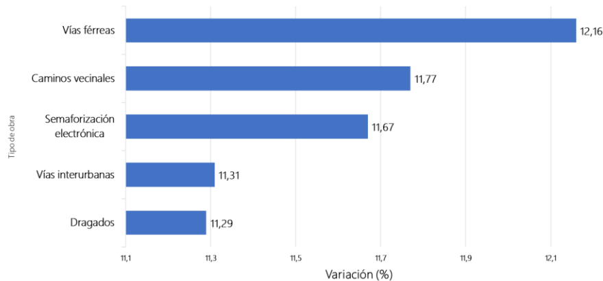
Gráfica 6. ICOCIV. Mayores variaciones anuales, según tipología de obra Total nacional Octubre 2023
