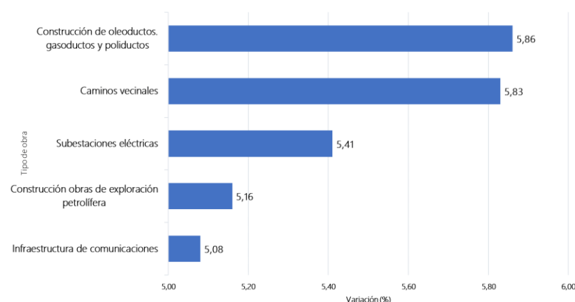
Gráfica 6. ICOCIV. Mayores variaciones anuales, según tipología de obra Total nacional Septiembre 2024
