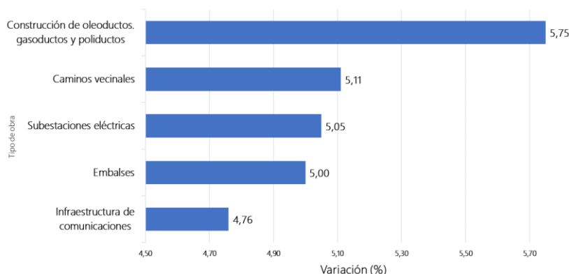
Gráfica 4. ICOCIV. Mayores variaciones del año corrido, según tipología de obra Total nacional Septiembre 2024
