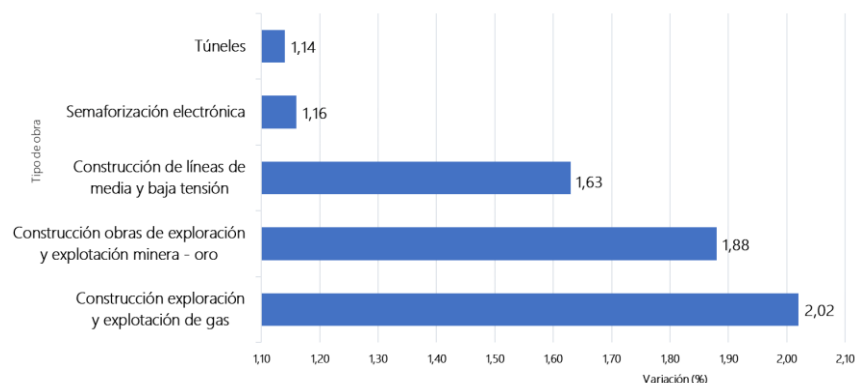
Gráfica 7. ICOCIV. Menores variaciones anuales, según tipología de obra Total nacional Septiembre 2024
