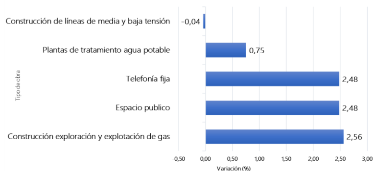
Gráfico 5. ICOCIV. Menores variaciones del año corrido, según tipología de obra Total nacional Septiembre 2025
