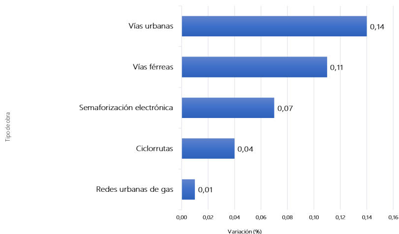
Gráfico 3. ICOCIV. Mayores variaciones mensuales positivas, según tipología de obra Total nacional Septiembre 2025
