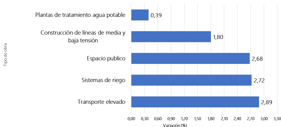
Gráfico 7. ICOCIV. Menores variaciones anuales, según tipología de obra Total nacional Septiembre 2025
