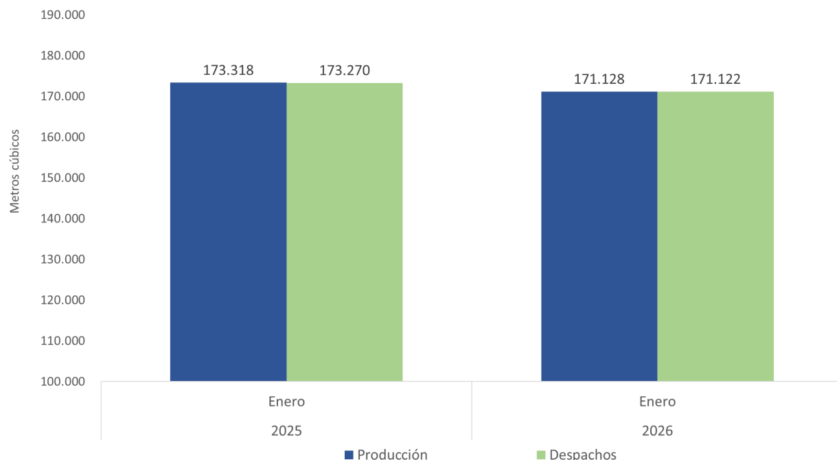
Gráfico 1. Producción y despachos de mezcla asfáltica (metros cúbicos) Total nacional Enero (2025-2026) pr
